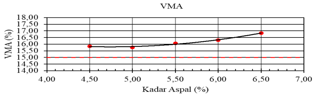
Gambar 4. Hubungan Kadar aspal dengan VMA
