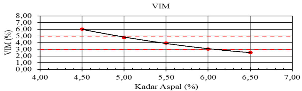
Gambar 5. Hubungan Kadar Aspal dengan VIM
