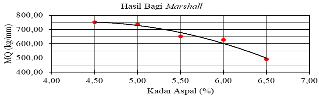
Gambar 7. Hubungan Kadar Aspal dengan Hasil Bagi Marshall
