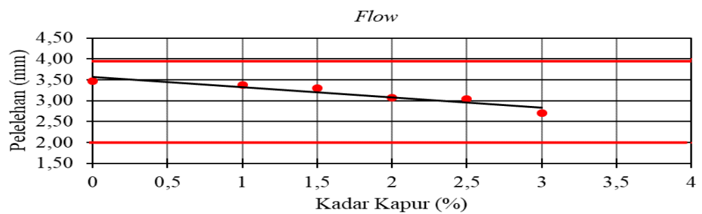
Gambar 14. Hubungan Variasi Kapur Terhadap Flow
