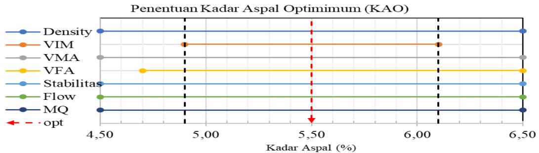
Gambar 8. Penentuan Kadar Aspal Optimum
