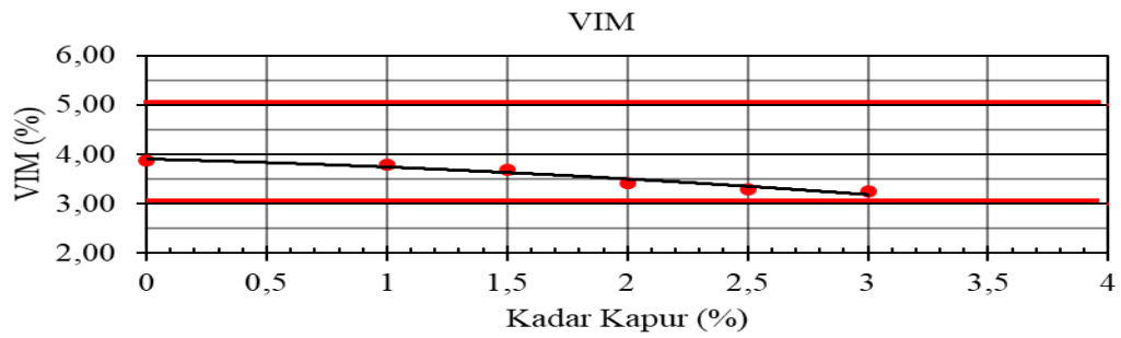
Gambar 10. Hubungan Variasi Kapur Terhadap VIM
