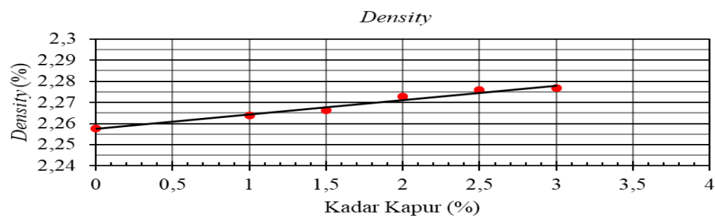
Gambar 9. Hubungan Variasi Kapur Terhadap Density
