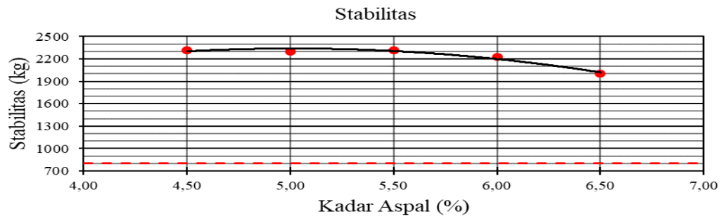
Gambar 2. Hubungan Kadar Aspal dengan Stabilitas
