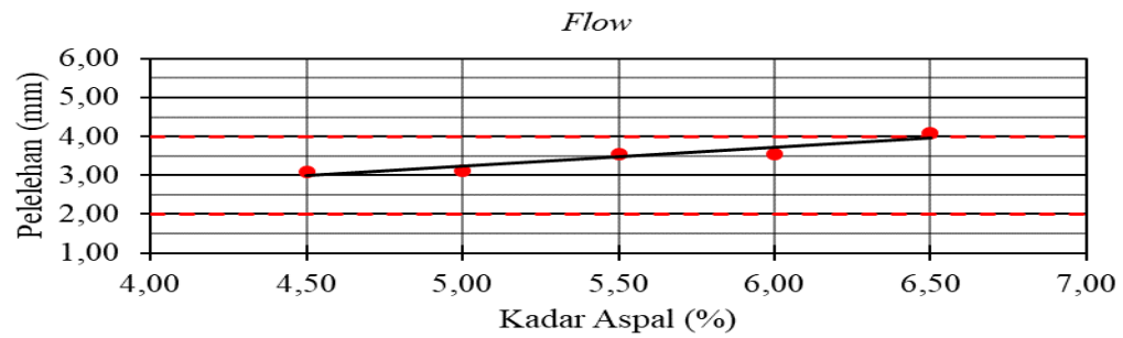
Gambar 3. Hubungan Kadar Aspal dengan Flow
