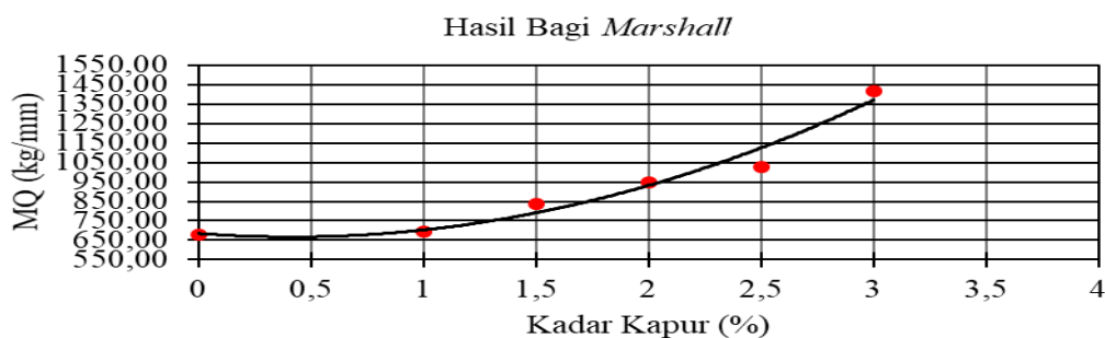
Gambar 15. Hubungan Variasi Kapur Terhadap Hasil Bagi Marshall
