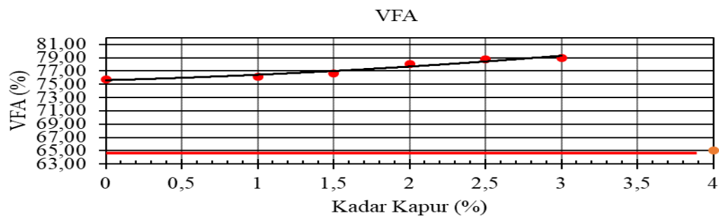
Gambar 12. Grafik Hubungan Variasi Kapur Terhadap VFA
