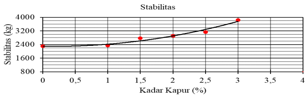
Gambar 13. Hubungan Variasi Kapur Terhadap Stabilitas
