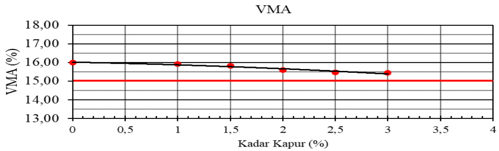
Gambar 11. Hubungan Variasi Kapur Terhadap VMA
